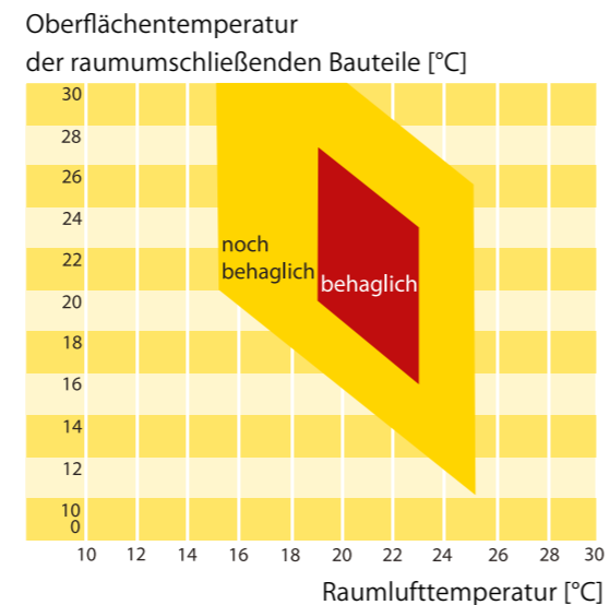
Abb. 4 | Abhängigkeit der thermischen Behaglichkeit von der Wand-Oberflächentemperatur
