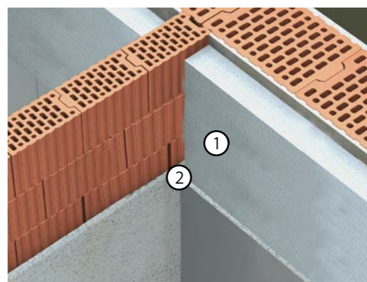
Abb. 12 | Innendämmung
