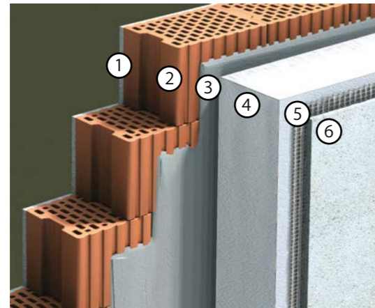
Abb. 8 | Wärmedämmverbundsystem
