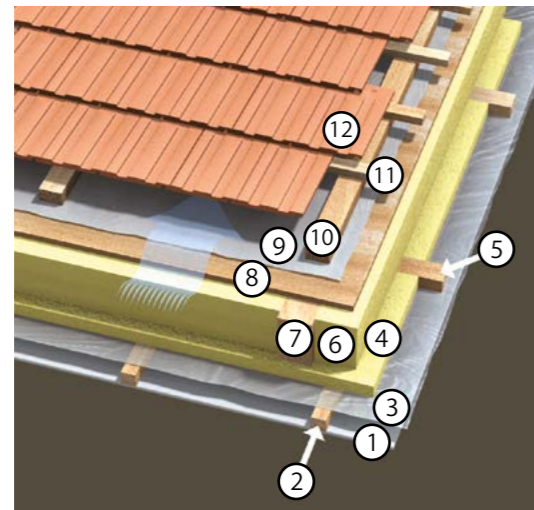
Abb. 14 | Zwischensparrendämmung
