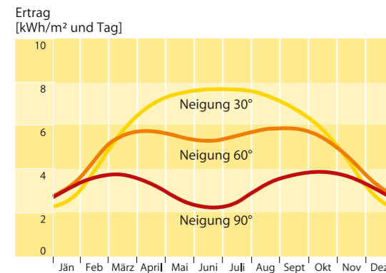
Abb. 38 | Ertrag der Kollektoren bei unterschiedlicher Neigung
