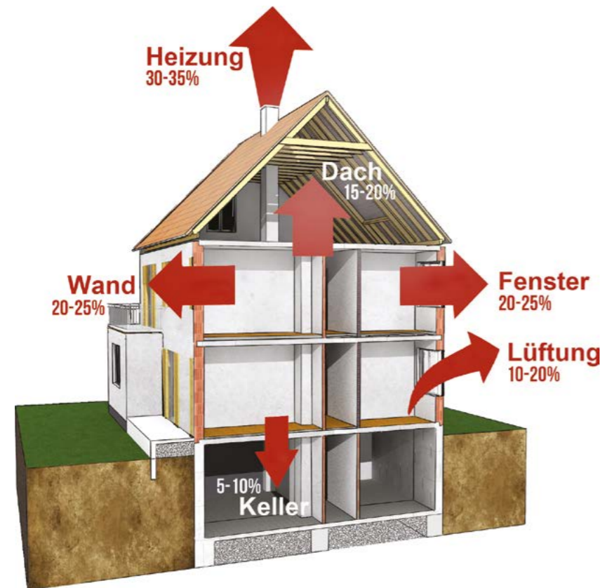
Abb. 1 | Energieverluste über verschiedene Bauteile
