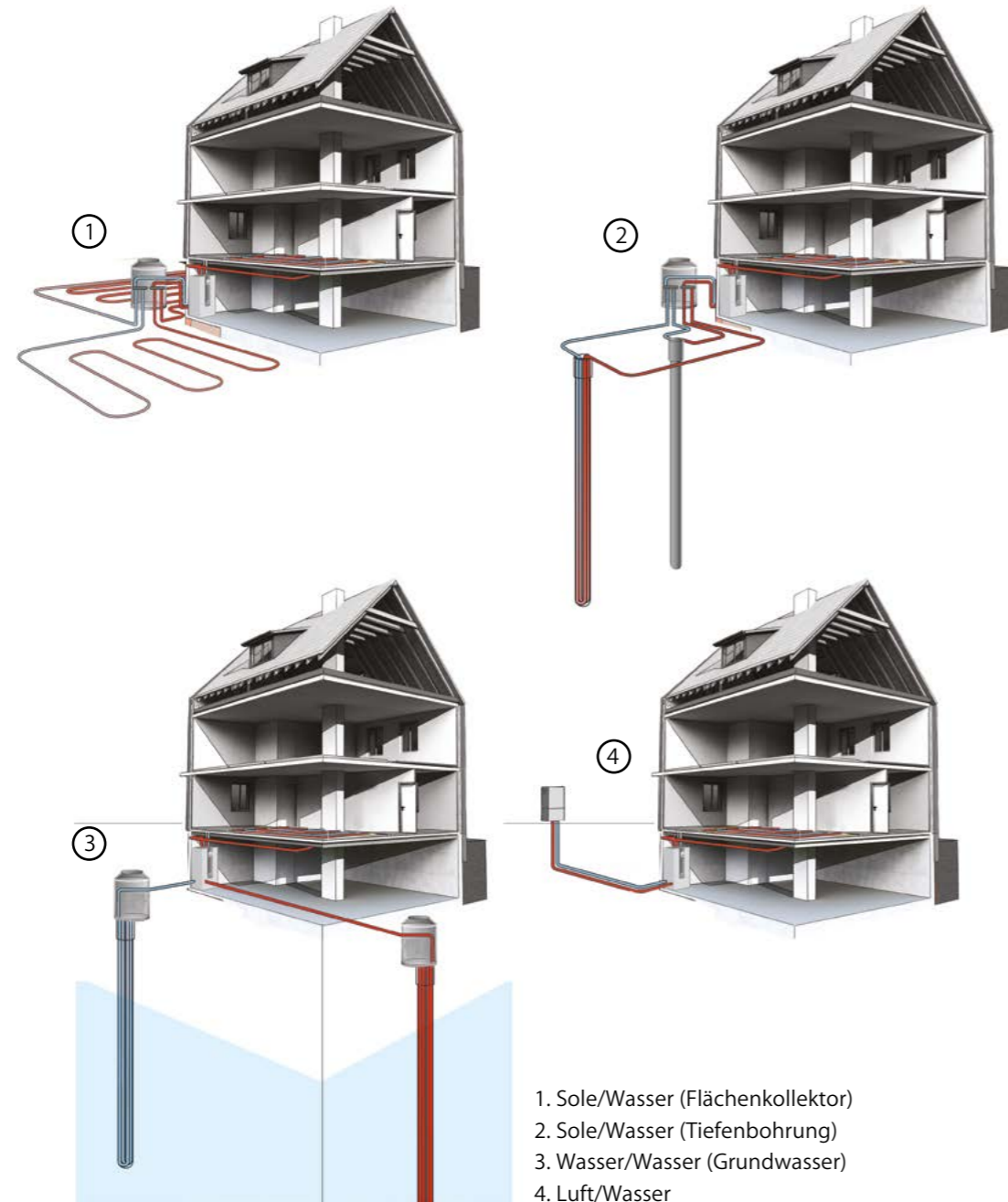
Abb. 30 | Wärmepumpentypen
