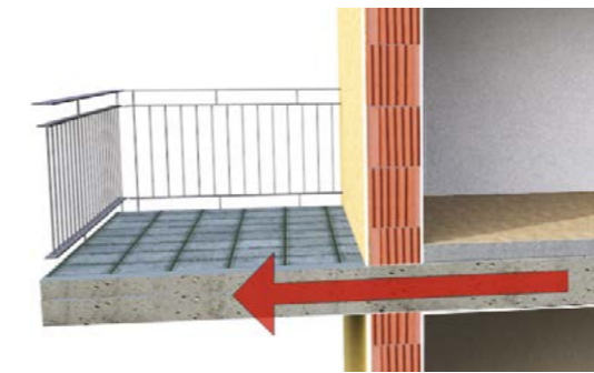
Abb. 24 | Massive Wärmebrücke: Durchgehend betonierte Balkonplatte
