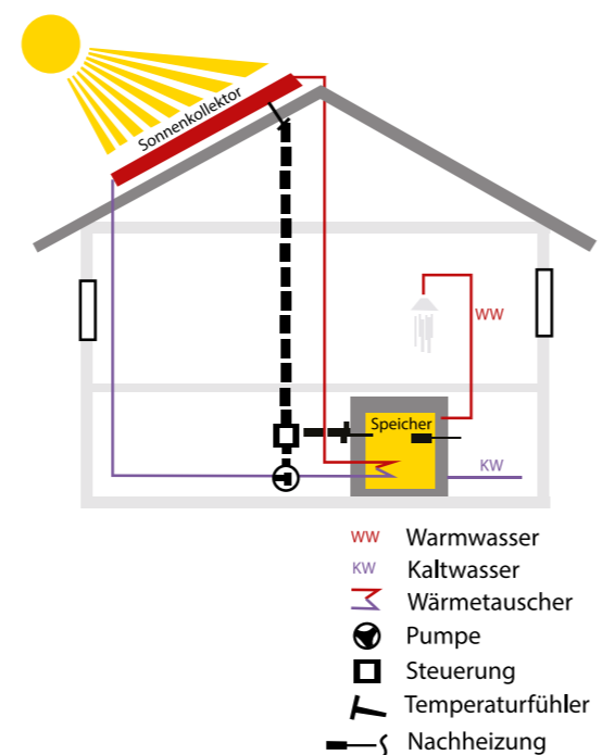
Abb. 42 | Anlagenschema: Solare Warmwasserbereitung
