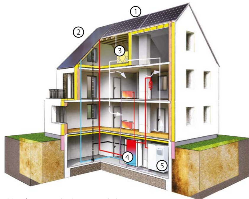
Abb. 27 | Saniertes Gebäude mit Haustechnik
