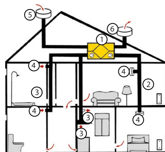
Abb. 43 | Kontrollierte Wohnraumlüftung, Zu- und Abluftanlage
