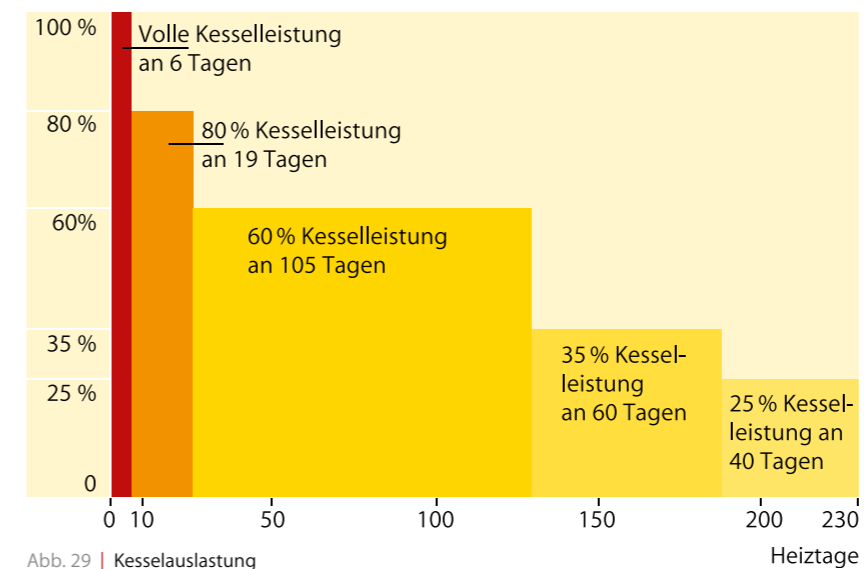
Abb. 29 | Kesselauslastung
