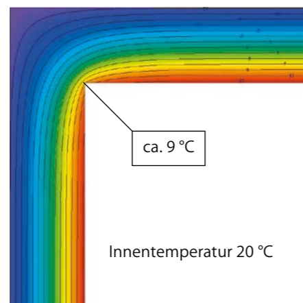
Abb. 23 | Oberflächentemperaturen von Außenecken – ohne und mit Dämmung
