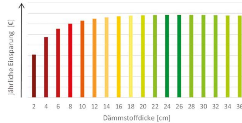
Abb. 6 | Kostenoptimale Dämmstoffstärke
