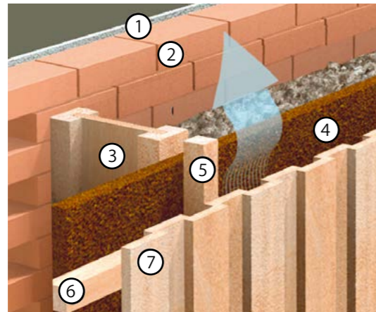
Abb. 11 | Hinterlüftete Fassade
